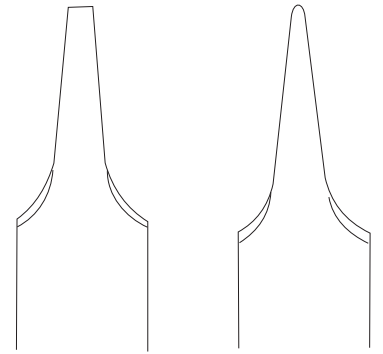
SB-2010-17 17 mm SB-2010-18 18 mm
